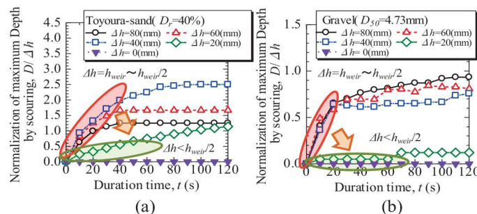
図-4 無次元最大洗堀深: (a)豊浦砂, (b)礫材
