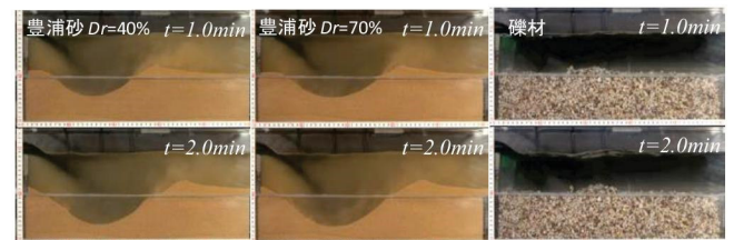
図-2 越流による洗堀現象の様子
