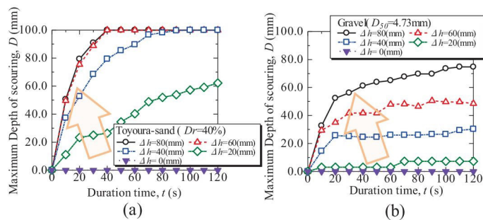
図-3 最大洗堀深: (a)豊浦砂, (b)礫材
