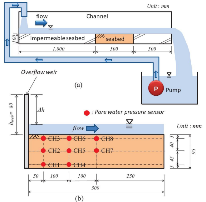
図-1 実験装置の模式図(a)および間隙水圧計の配置(b)
