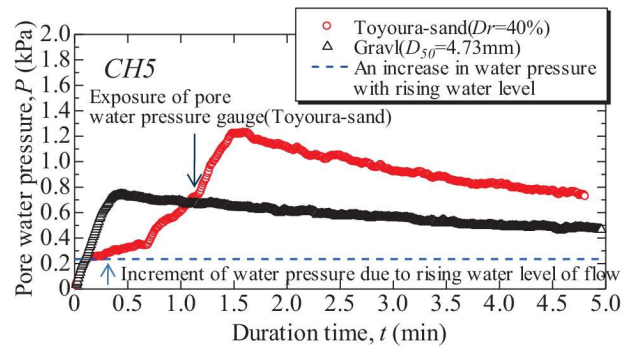
図-5 CH5における間隙水圧の時刻変化
