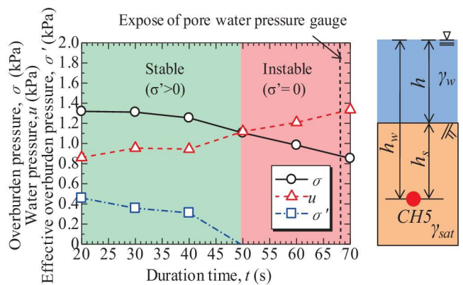
図-6 地盤内部の応力変化
