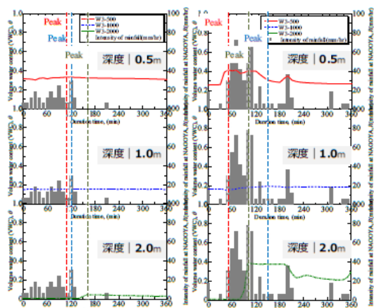
図 3-3 実堤防法面 (W3) の水分量変化 (左: 降雨強度 30mm/hr (台風相当), 右: 降雨強度 80mm/hr (集中豪雨相当))
