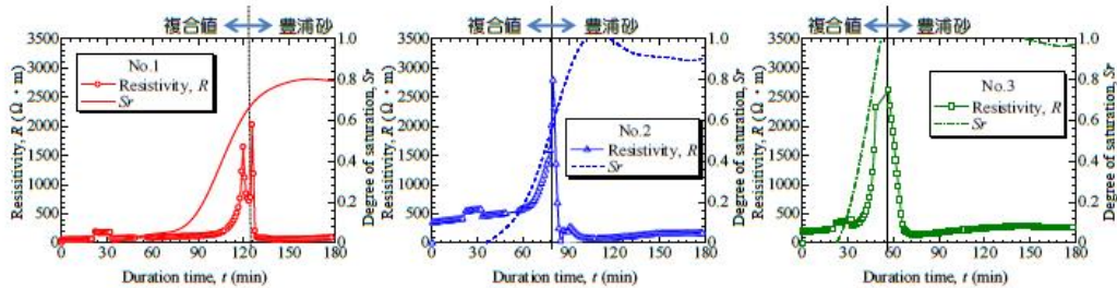
図 4-6 Case9 における比抵抗値・水分量の時刻歴：左図は計測器位置 No.1 (土槽底面から 150mm)、中央図は No.2 (底面から 100mm)、右図は No.3 (底面から 50mm) を示す。また、図中の黒点線より後が豊浦砂の比抵抗値を示す。
