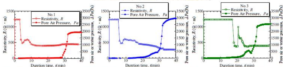
図 4-4 Case1 における比抵抗値と間隙空気圧の時刻歴: 左図は計測器位置 No.1 (土槽底面から 150mm), 中央図は No.2 (底面から 100mm), 右図は No.3 (底面から 50mm) における時刻歴を示す。
