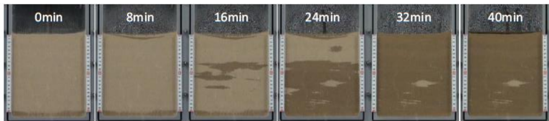
図 4-2 乾燥地盤へ集中豪雨に相当する降雨強度 135mm/hr を与えた際の浸潤及び浸透過程の時刻歴 (Case1)
