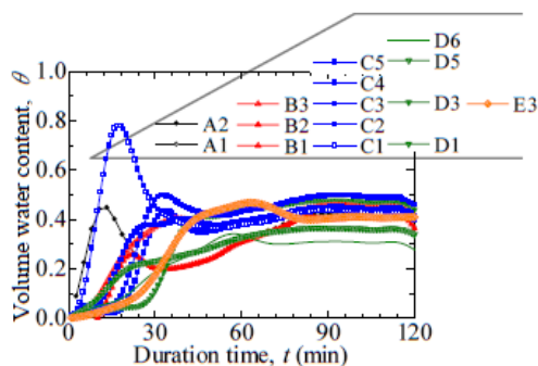
図 2-7 降雨強度 80mm/hr 時 (猛烈な雨), 雨滴大における水分量比較
