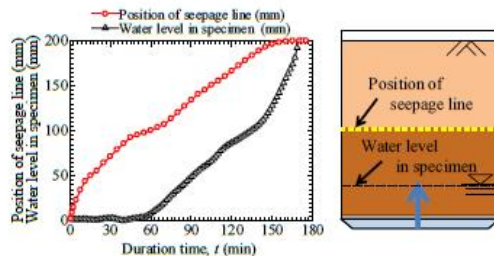
図 4-7 Case9 における浸潤線のフロントの位置と地盤内水位の時刻歴
