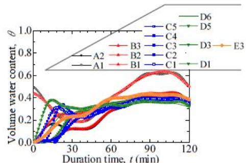
図 2-6 降雨強度 80mm/hr 時（猛烈な雨），雨滴小における水分量変化
