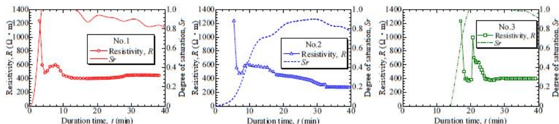
図 4-3 Case1 における比抵抗値・水分量の時刻歴: 左図は計測器位置 No.1 (土槽底面から 150mm), 中央図は No.2 (底面から 100mm), 右図は No.3 (底面から 50mm) における時刻歴を示す。
