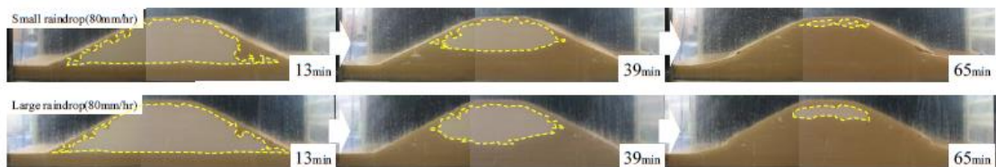
図 2-3 降雨強度 80mm/hr 時（猛烈な雨）における堤体断面の比較，上：雨滴小，下：雨滴大
