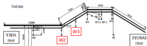
図 3-1 実堤防水分計埋設地点図
