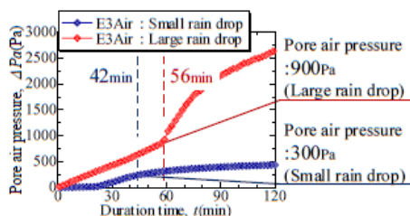
図 2-9 雨滴径の違いによる間隙空気圧変化の比較
