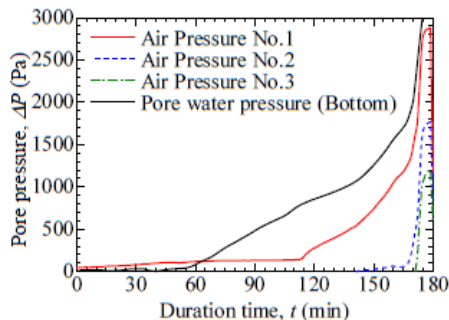
図 4-8 Case9: 各深度の間隙空気圧時刻歴
