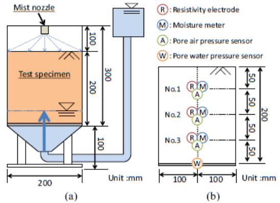
図 4-1 実験装置の概略図(a): 実験装置全体図, (b): 地盤内の各計測器の設置位置
