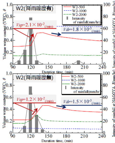
図 3-4 降雨強度 80mm/hr 時 (集中豪雨相当) の実堤防内浸潤及び排水速度比較 (上: 降雨履歴有, 下: 降雨履歴無)
