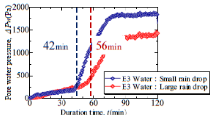
図 2-8 雨滴径の違いによる間隙水圧変化の比較
