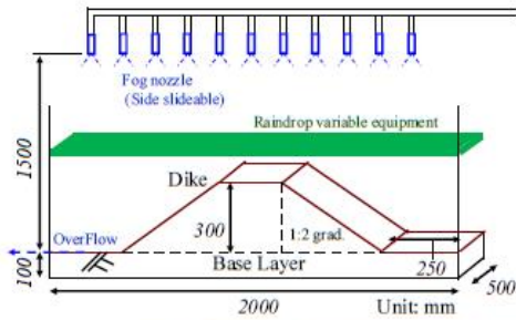
図 2-1 模型堤防試験装置概要
