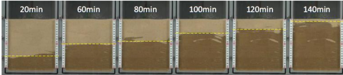
図 4-5 乾燥地盤へ降雨強度 30mm/hr に相当する流量を土槽底面から与えた際の浸潤及び浸透過程の時刻歴 (Case9)
