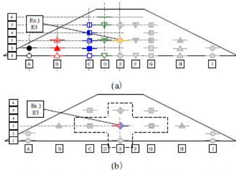
図 2-2 計測器埋設位置(a)：水分計，(b)：間隙水圧計，間隙空気圧計（黒点線内の位置）
