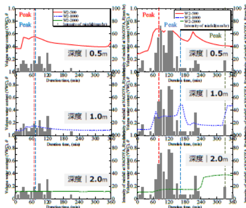
図 3-2 実堤防法面 (W2) の水分量変化 (左: 降雨強度 30mm/hr (台風相当), 右: 降雨強度 80mm/hr (集中豪雨相当))
